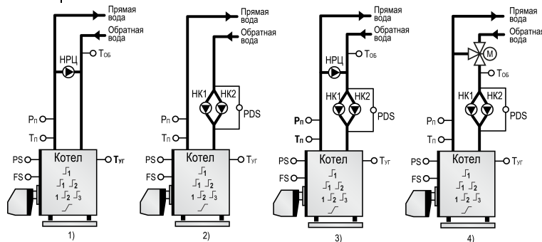
Рисунок 6.1 – Объект управления
